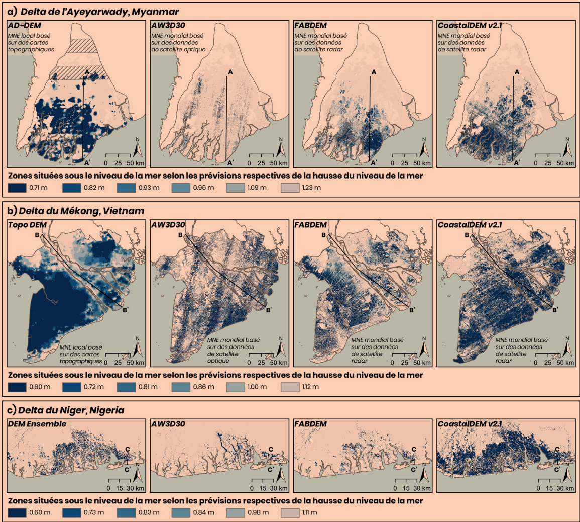
Figure 2 – Zone située sous le futur niveau moyen de la mer d'après les MNE locaux et mondiaux (a) Seeger et al. , 2023 ; b) Minderhoud et al. , 2019 (modifié) ; c) Hauser et al. , 2023).
