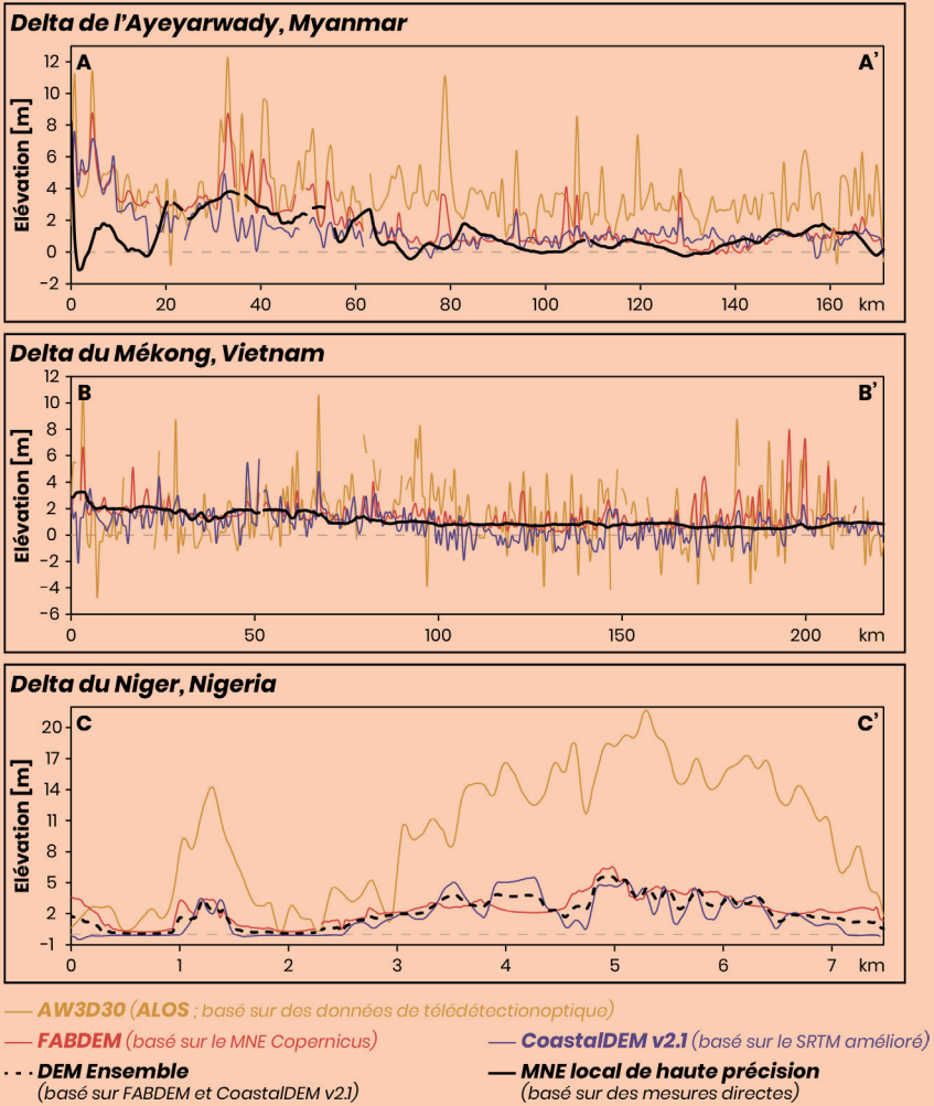
Figure 1 – Comparaison de MNE pour des zones côtières où l'on manque de données, sur la base des profils d'élévation
